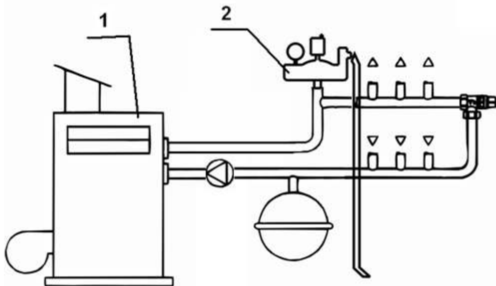
1 – Отопительный котел; 2 – Группа безопасности.
